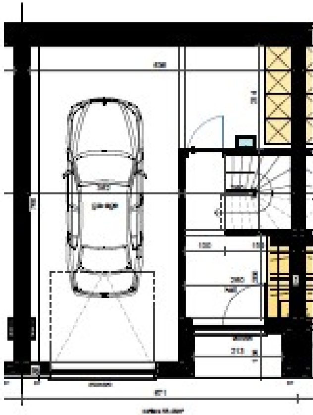
sous-sol 1:100
